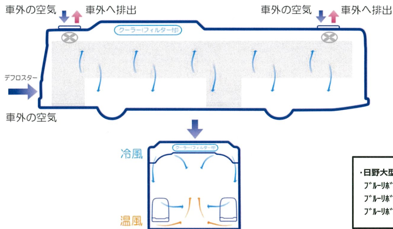
日野ブルーリボン 車内空調イメージ図
