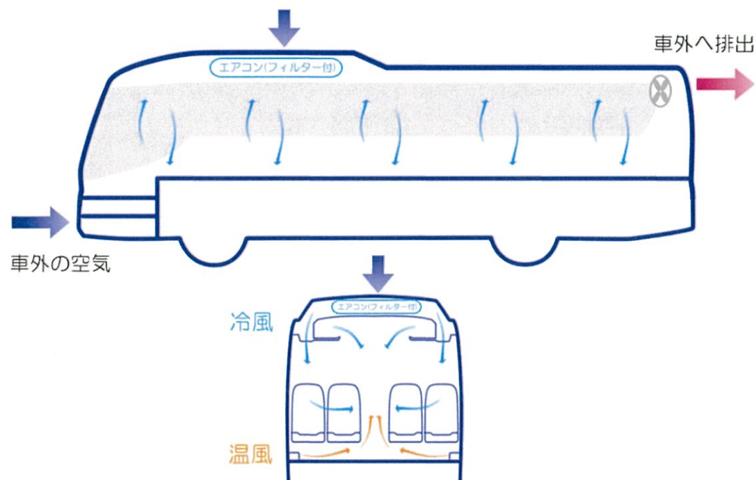
日野セレガ 車内空調イメージ図
